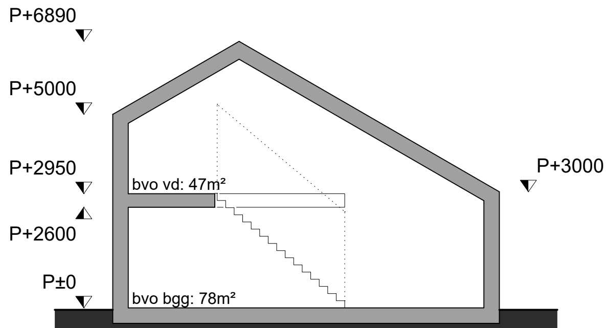
doorsnede woning 2
