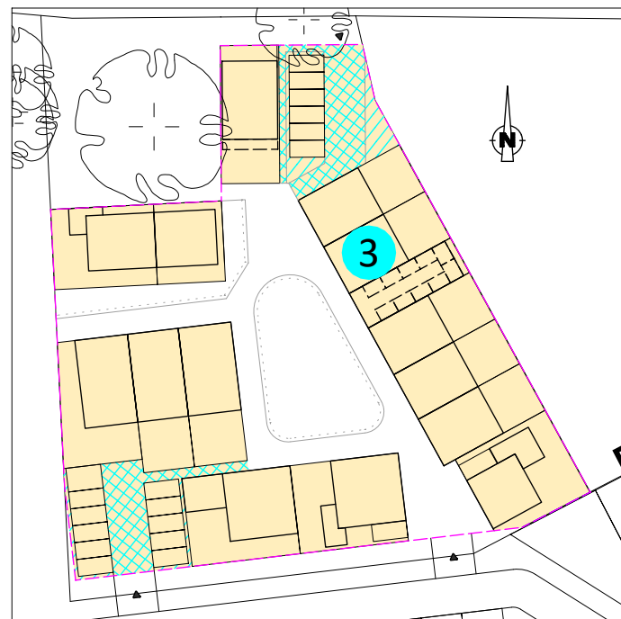
situatie 1:1000
