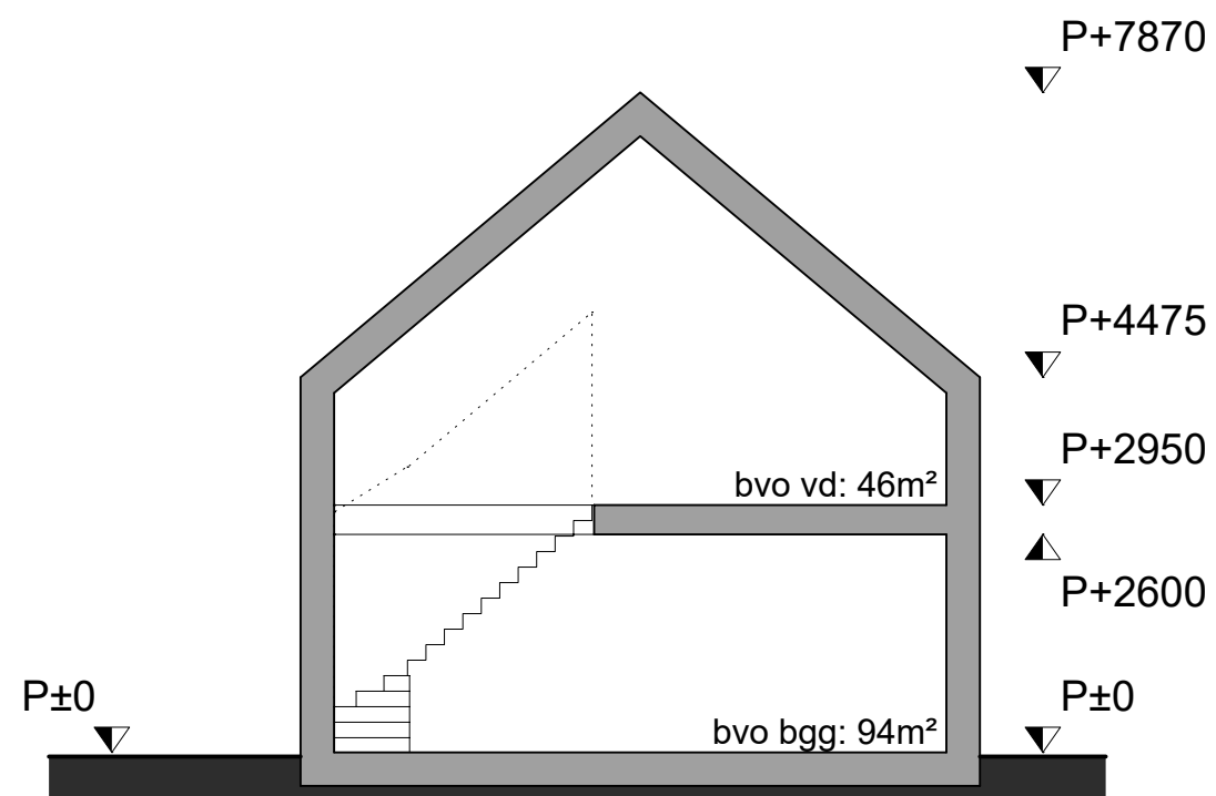
doorsnede woning 1
