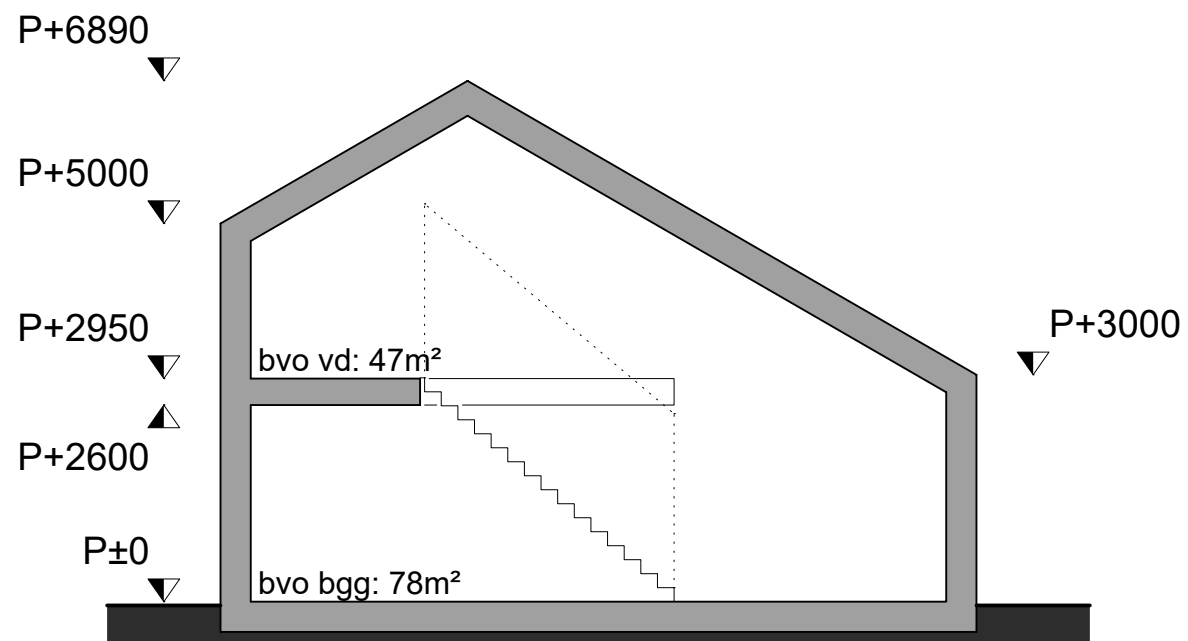
doorsnede woning 6
