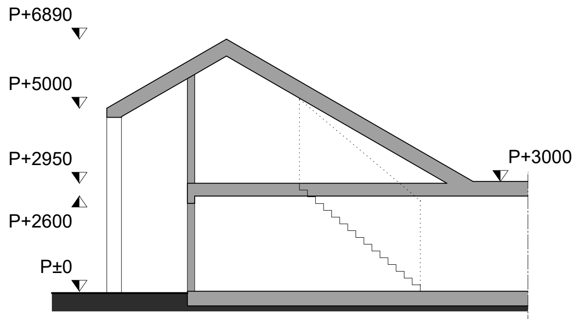
doorsnede bergingen
