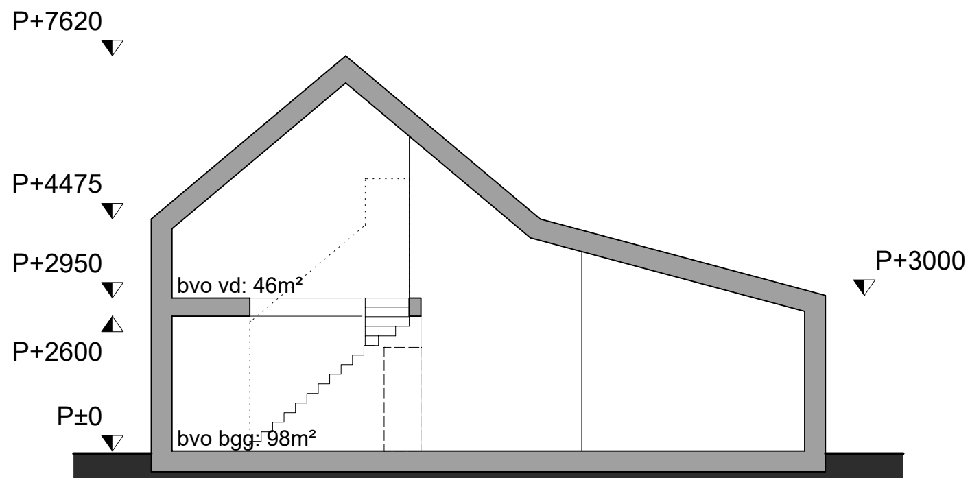
doorsnede woning 11
