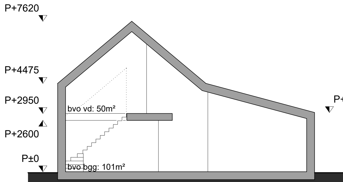
doorsnede woning 12
