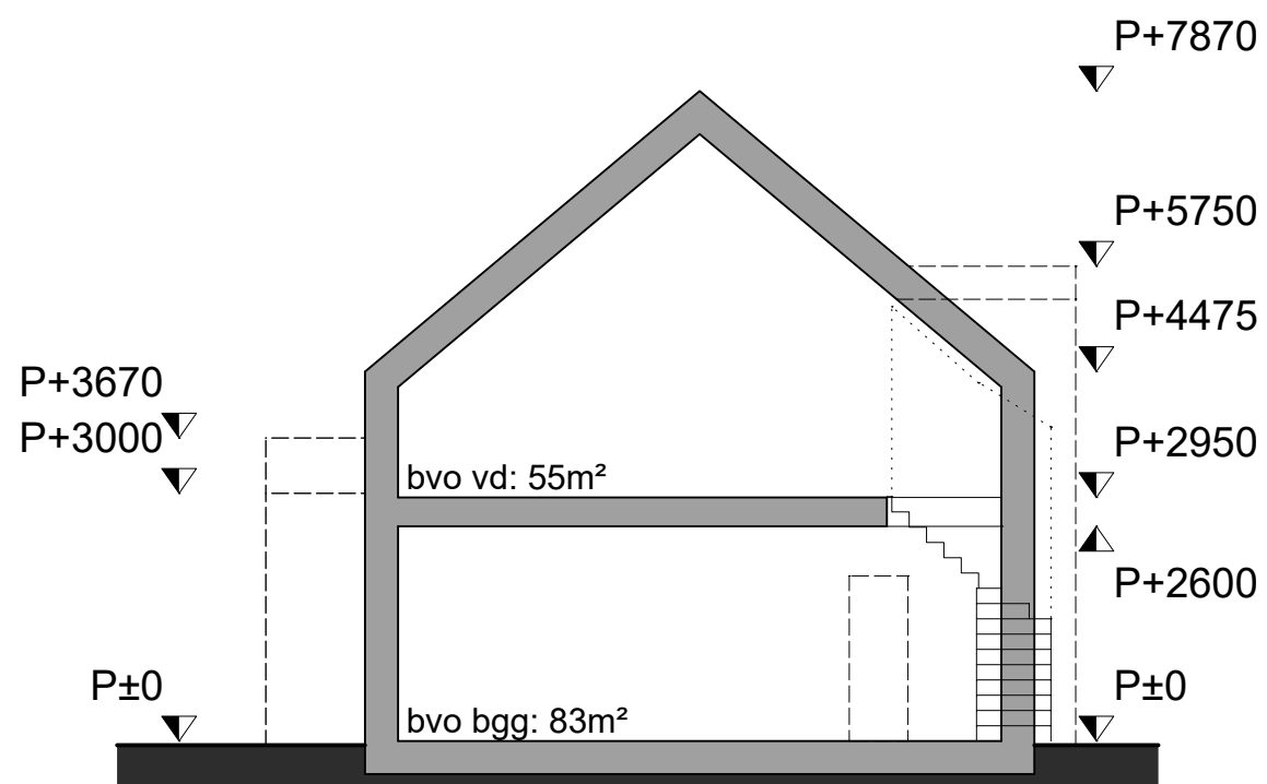
doorsnede woning 13
