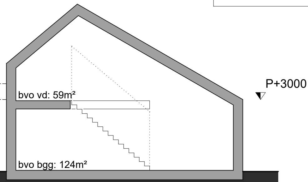
doorsnede woning 9
