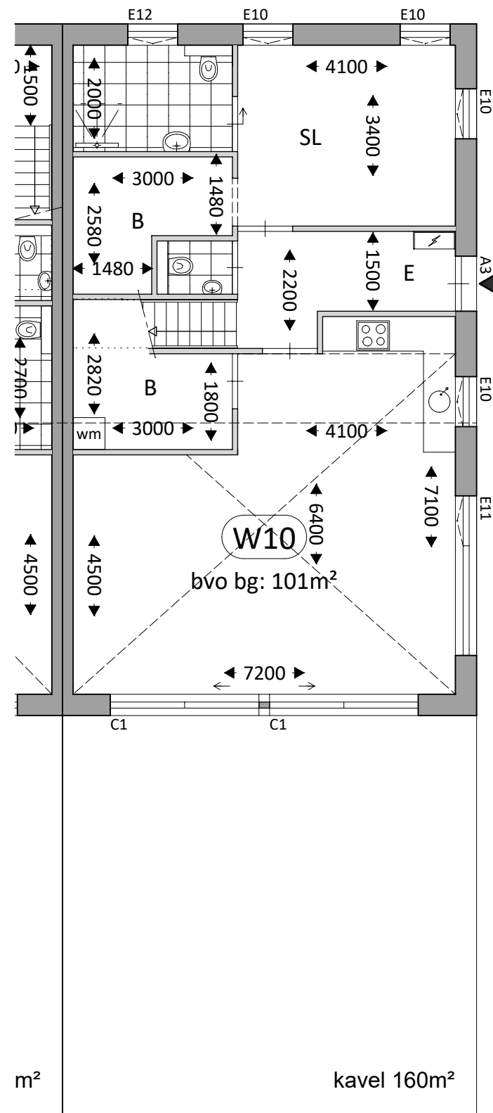
begane grond
