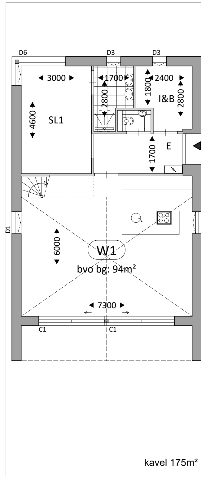
begane grond
