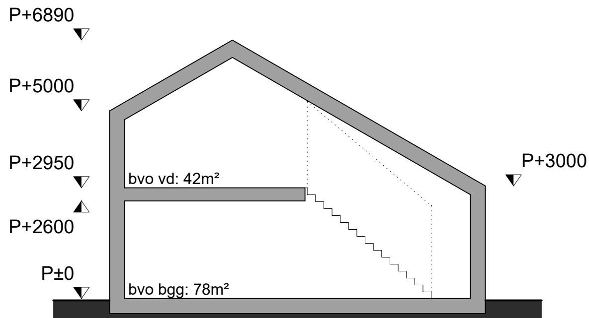
doorsnede woning 4
