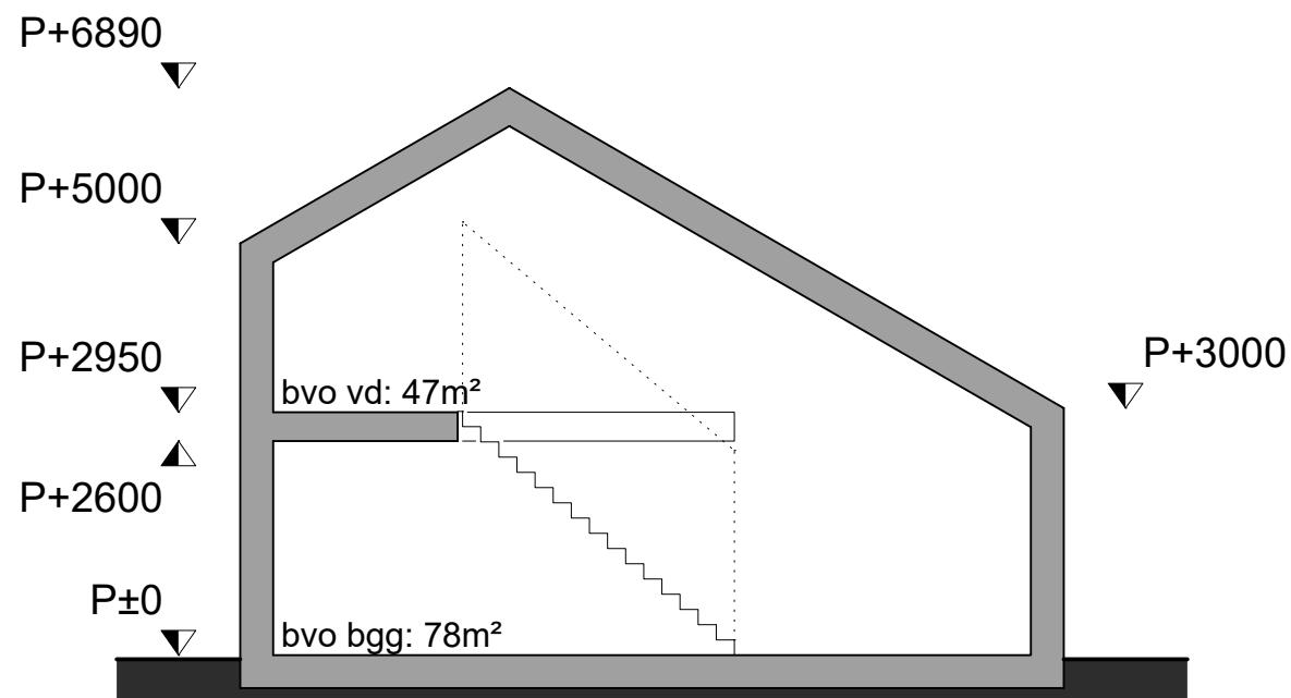
doorsnede woning 3
