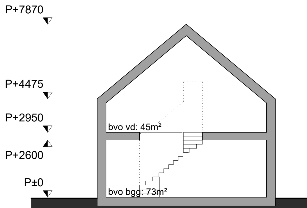
doorsnede gemeenschappelijk
