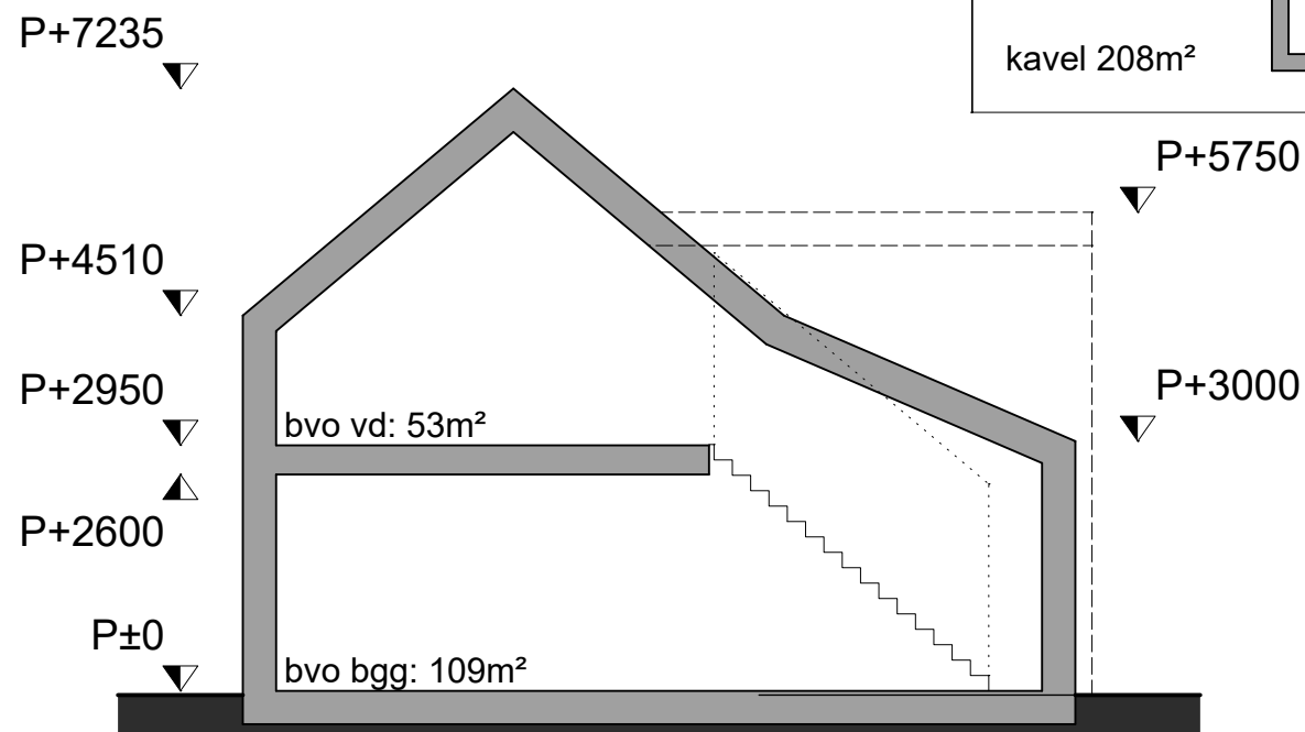
doorsnede woning 8
