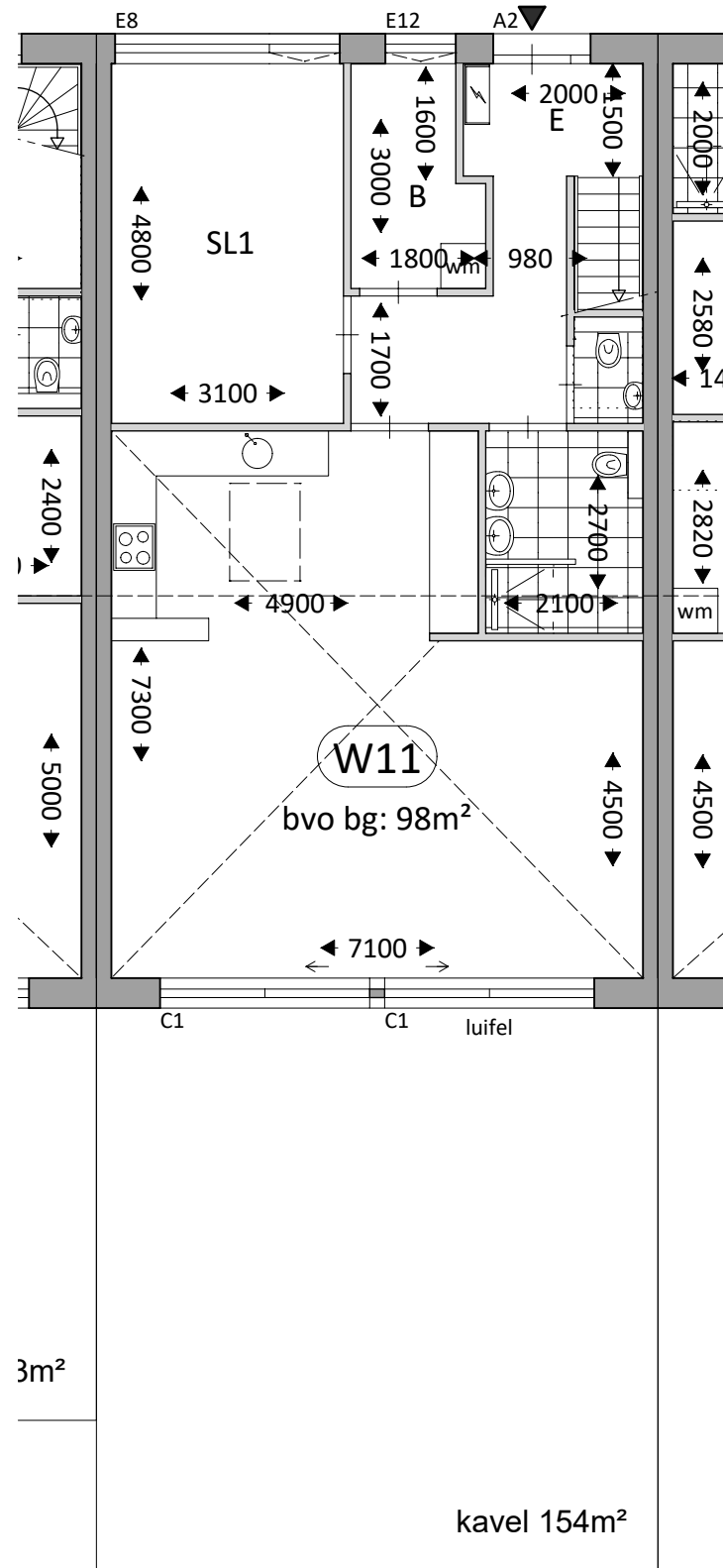
begane grond
