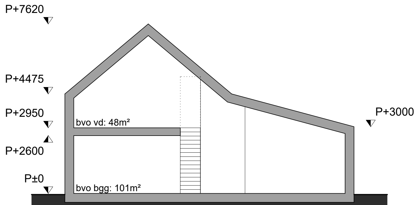
doorsnede woning 10
