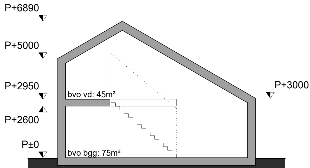
doorsnede woning 5
