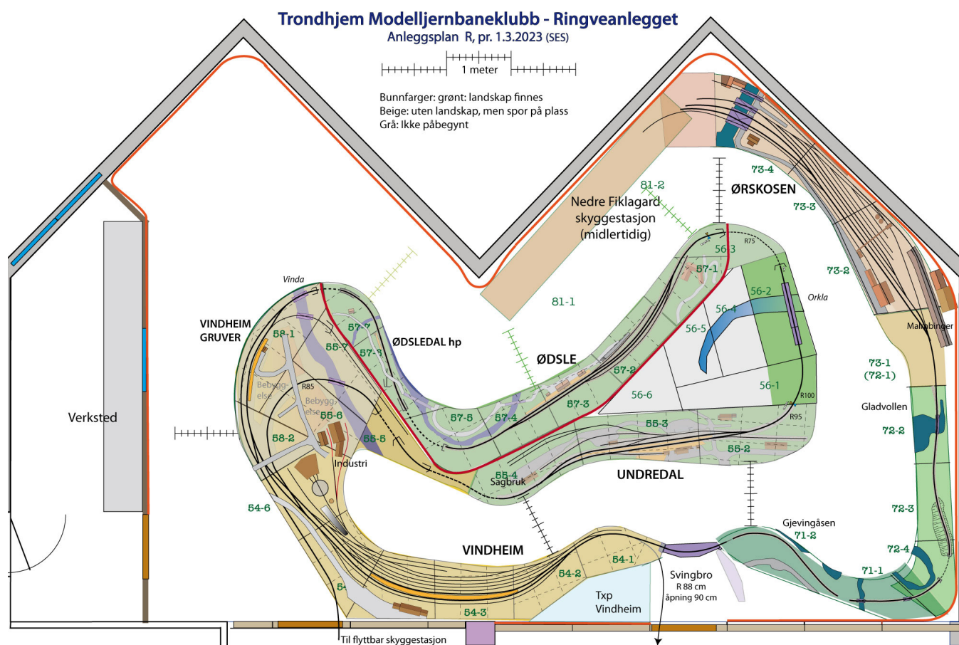
Fig. 1 - Plan over anlegget ved starten av 2023
