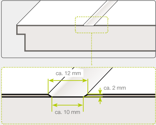
Lines Art | Querschnitt
