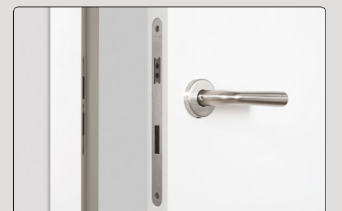
Das Schließblech ist bei geschlossener Tür nicht sichtbar, da das Schloss magnetisch verriegelt wird, ohne mechanischen Kontakt zum Schließblech.
